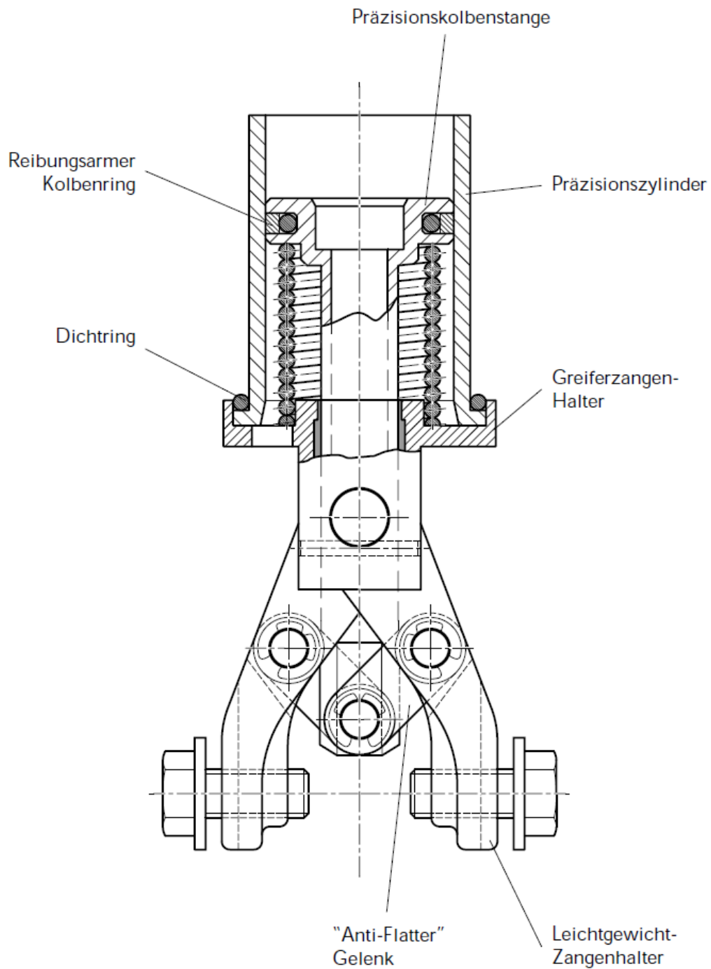
Greiferzangen-Halter 191-9535
